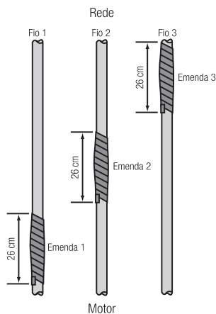
Figura 10: Posição das emendas
