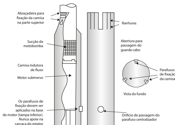
Figura 12: Detalhe da camisa indutora de fluxo
